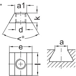
Muttern für V-Nuten 60° Festigkeitsklasse 10
