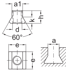
Muttern für V-Nuten 60° Festigkeitsklasse 10
