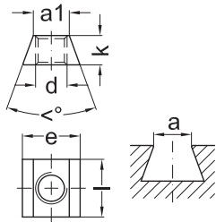
Muttern für V-Nuten 40° Festigkeitsklasse 10
